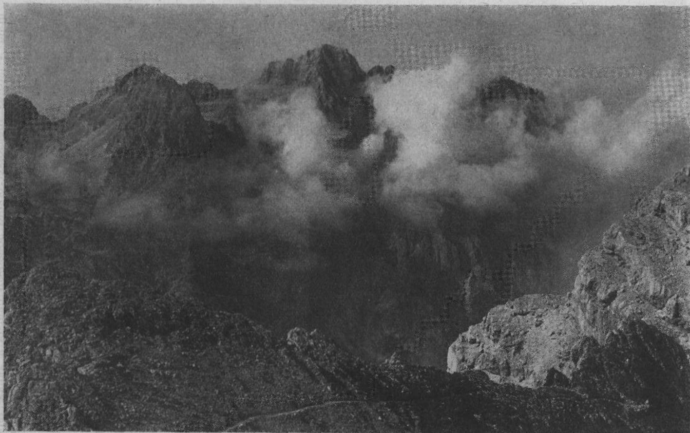
Slika 4. Toplotne megle ob pobočjih Škrlatice
