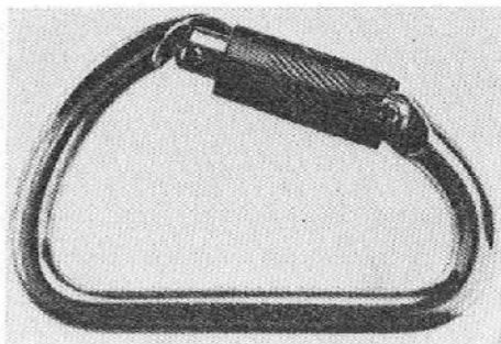
Na sliki je vponka tipa TL (Twist Lock) firme Elite. Skoraj vse firme, ki v Evropi izdelujejo vponke, ponujajo zdaj vsaka svojo varianto novega tipa vponke
