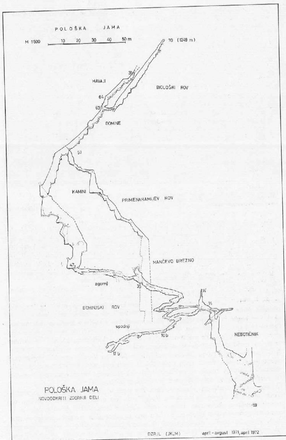
Načrt na nove odkritih delov v Pološki jami
