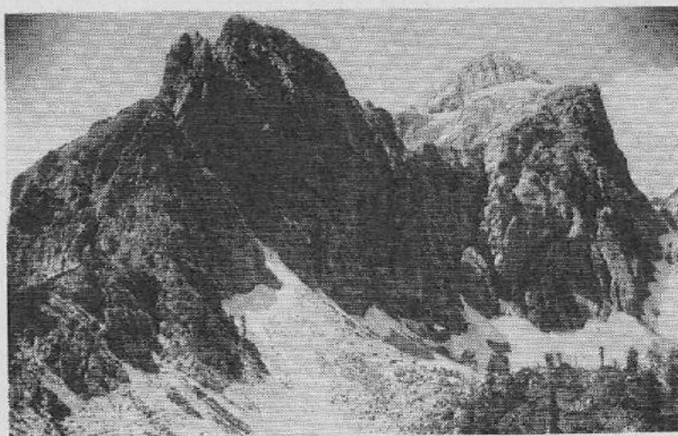
Grebeni Mojstrovke, polne škrbin, štrlekov in sipcev grintavca
