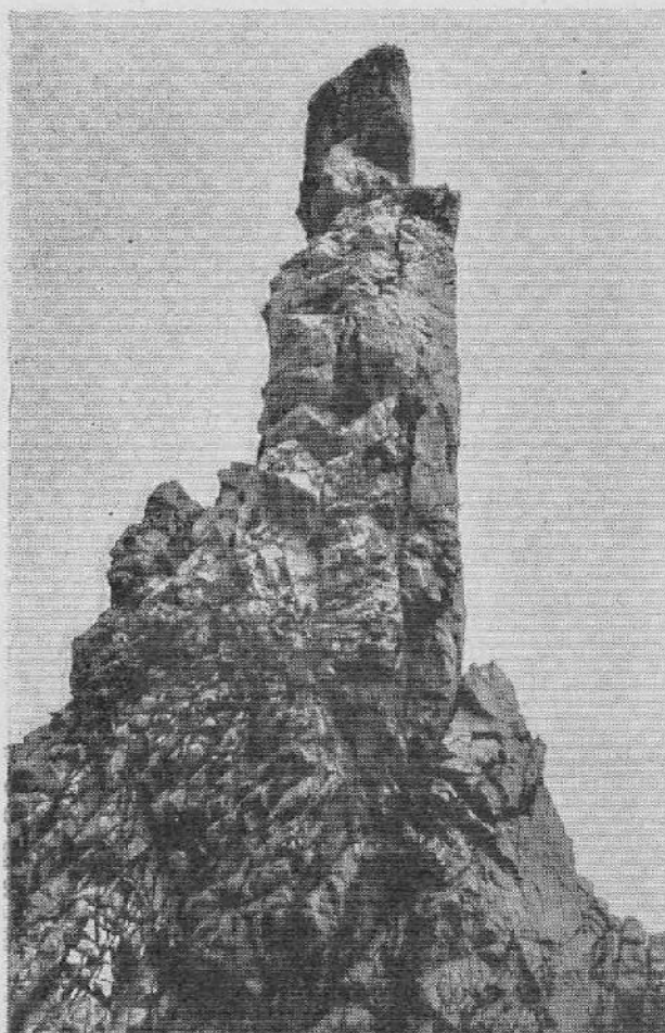
Dolomiti štrlek — Grintavi vrhovi, stene, grebeni so oškrbljeni, se koljejo, pokajo, razpadajo se drobijo in meljejo v robat grušč in oster drobni melišč
